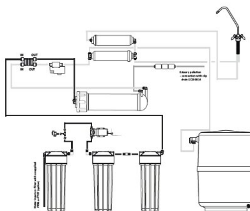
Model cu pompa Booster si cartus remineralizare
